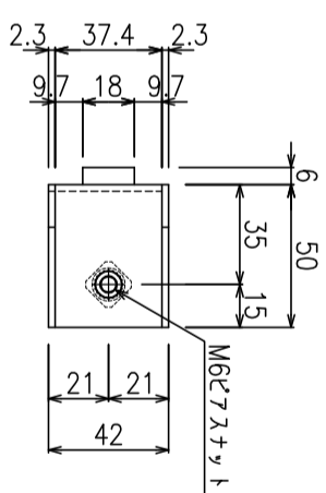
下綱線取付金具 S=1/2
